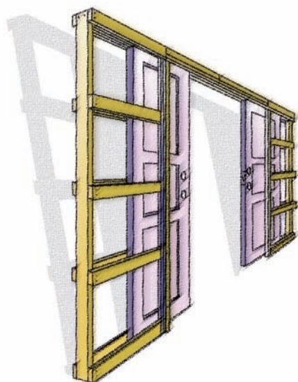
2-FLØYA SKYVEDØRSKARM
