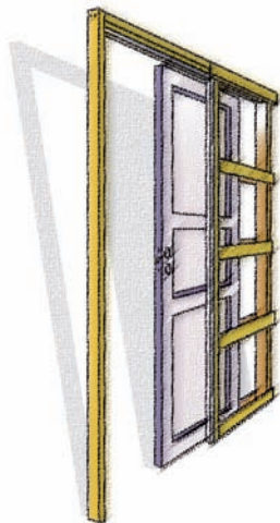
1-FLØYA SKYVEDØRSKARM
