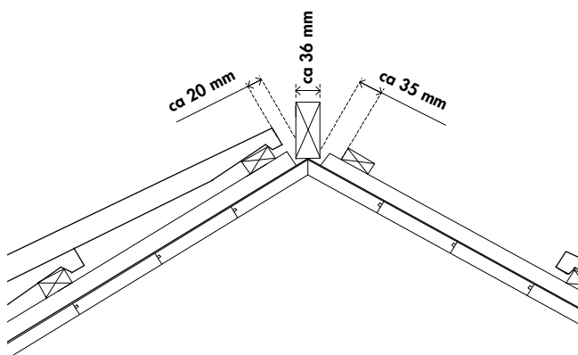
Bilde 4: Øverste bærelekten.
