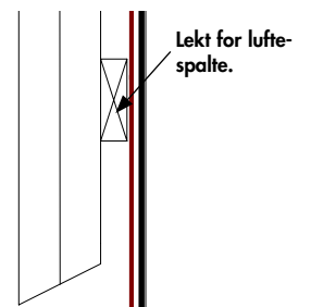
Bilde 7: Veggavslutning, montering av skjult avrenningsbeslag.
