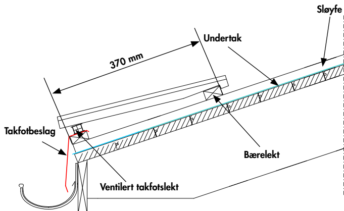
Bilde 2. Takfotsløsning.
