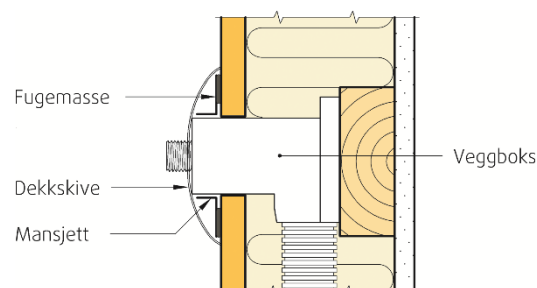
Fig. 3 Rørgjennomføring hvor mansjett limes fast til baderomspanelet
