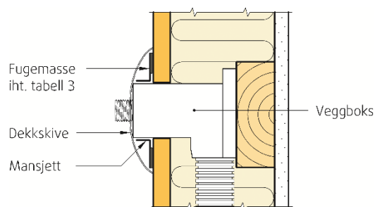
Fig. 3 Rørgjennomføring hvor mansjettens limes fast til baderomspanelet
