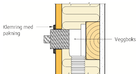
Fig. 4 Rørgjennomføring ved bruk av en tetningsring
