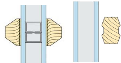
Pålimte sprosser
