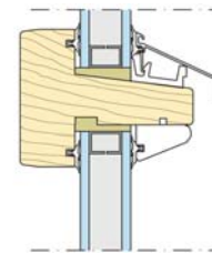
Gjennomgående sprosser
