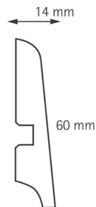
Sokkellist
