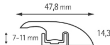
Nivålist
