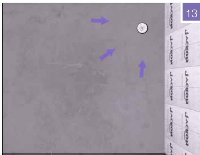
Fig. 13: Varmekabler (maksimalt 140 W/m 2 ) kan monteres direkte på våtromsplatene. Det er viktig å prime platene for god vedheft før avretting av gulv med flytstøp. Husk også å sørge for tilstrekkelig fall mot sluk.
