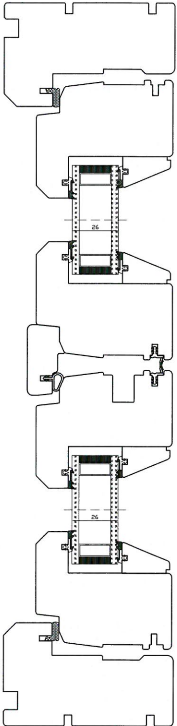
Tversnitt B
