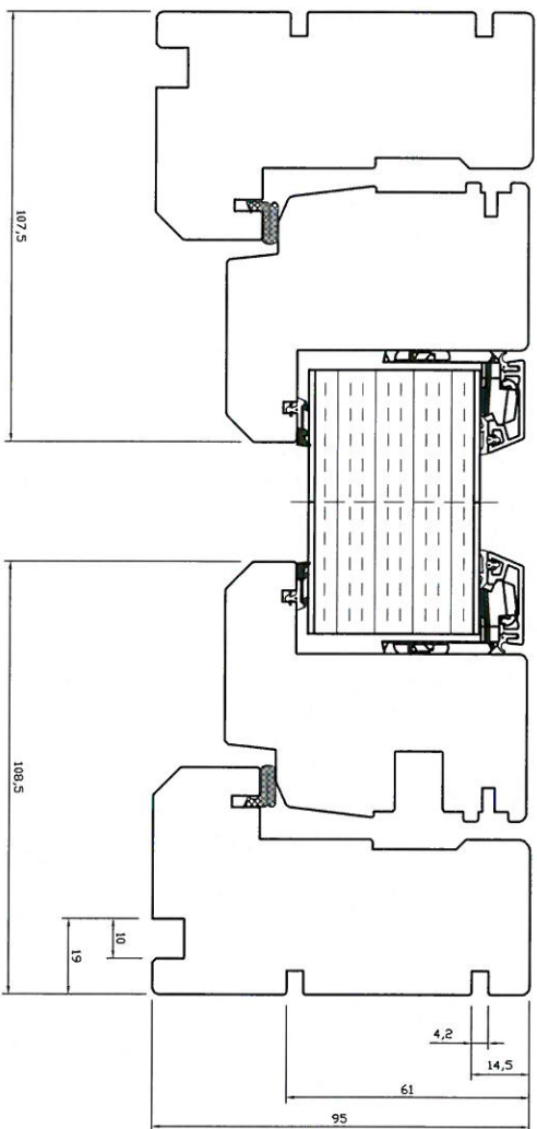
Tversnitt A
