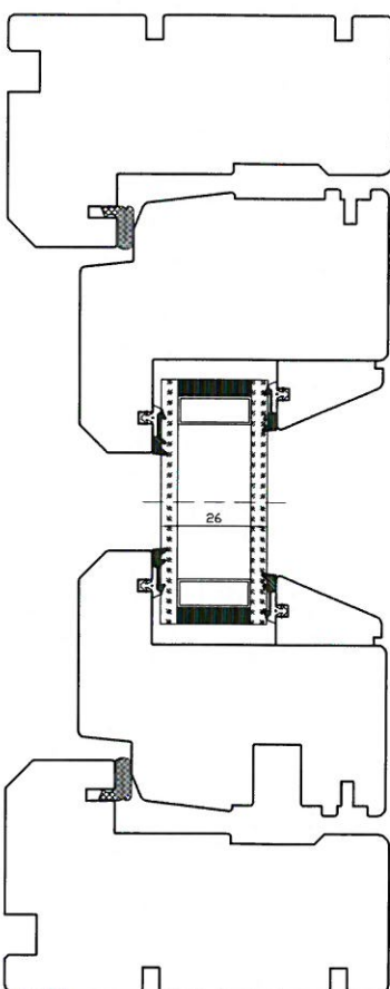
Tversnitt B
