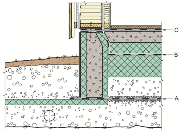
Fig. 1 Prinsipiell plassering av radonsperrer i ulike bruksgrupper. Jackon Radonsperre er godkjent i bruksgruppe B.
