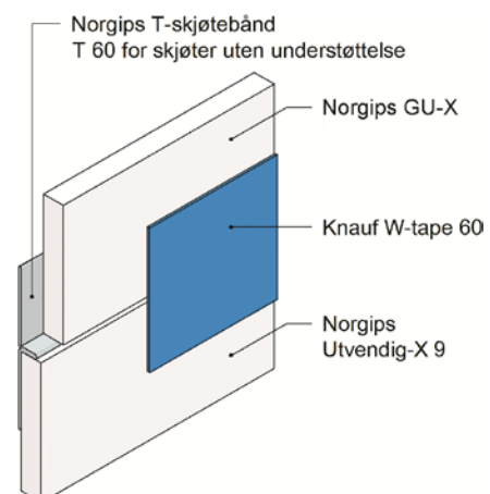
Fig.1b. Prinsipp for Norgips Vindtett System med Knauf W-tape og Norgips T-skjøtebånd T60.
