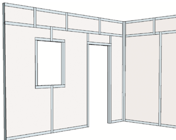
Fig. 8 Eksempel på bruk av Knauf W-tape til tetting av plateskjøter og rundt åpninger for dører og vinduer.
