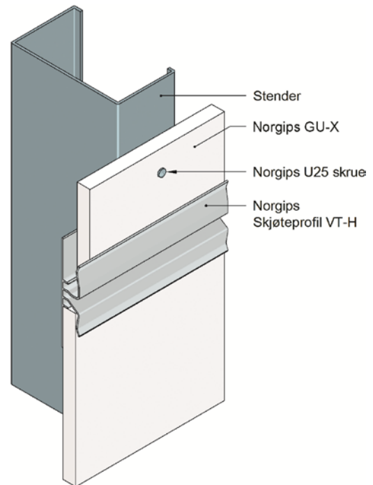
Fig.1a. Prinsipp for Norgips Vindtett System med Norgips horisontalt skjøteprofil VT-H.
