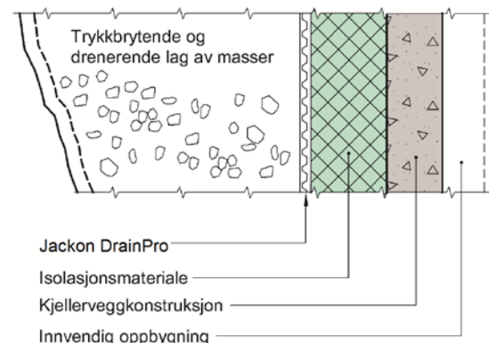
Fig. 2 Bruk av Jackon DrainPro på isolert vegg mot terreng. For raskere uttørring anbefales at Jackon DrainPro plasseres utenpå dampåpen varmeisolasjon som f.eks. EPS, se Byggforskserien 523.111 Yttervegger mot terreng. Varmeisolering og tetting.
