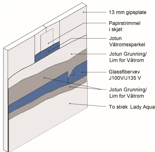
Fig. 1 Systemoppbygging for Lady Aqua på gipsplatekledning
